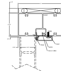
7B OPTIONAL NO TRANSOM DOOR HEAD
