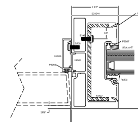
9 STANDARD HD INT. DOOR JAMB
