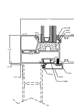
7 STANDARD DOOR HEADER
