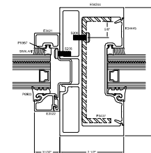
6 STANDARD HD TRANSOM JAMB
