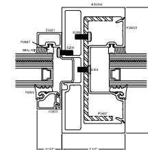
6A OPTIONAL HD DEEP POCKET TRANSOM JAMB
