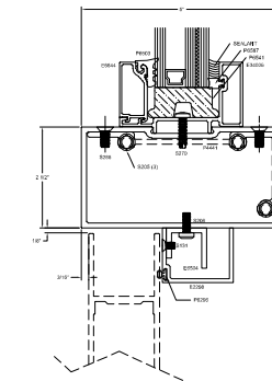
7A OPTIONAL DOOR HEADER
