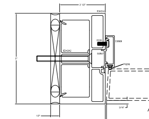
8A STANDARD HD DOOR JAMB
