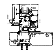
2B SILL SF ADAPTOR OPTIONAL
