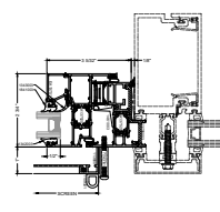
4A JAMB CURTAIN WALL INSTALLATION OPTIONAL
